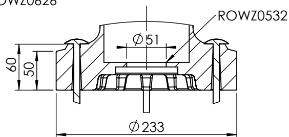
DETAIL B MAßSTAB 1 : 5
